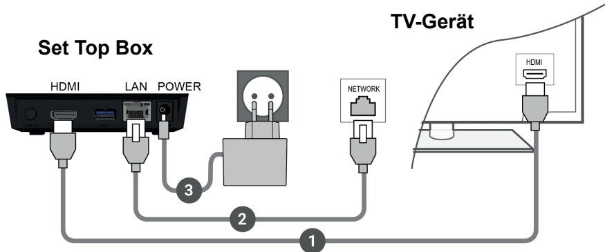
Abbildung 3: Kabelverbindungen
